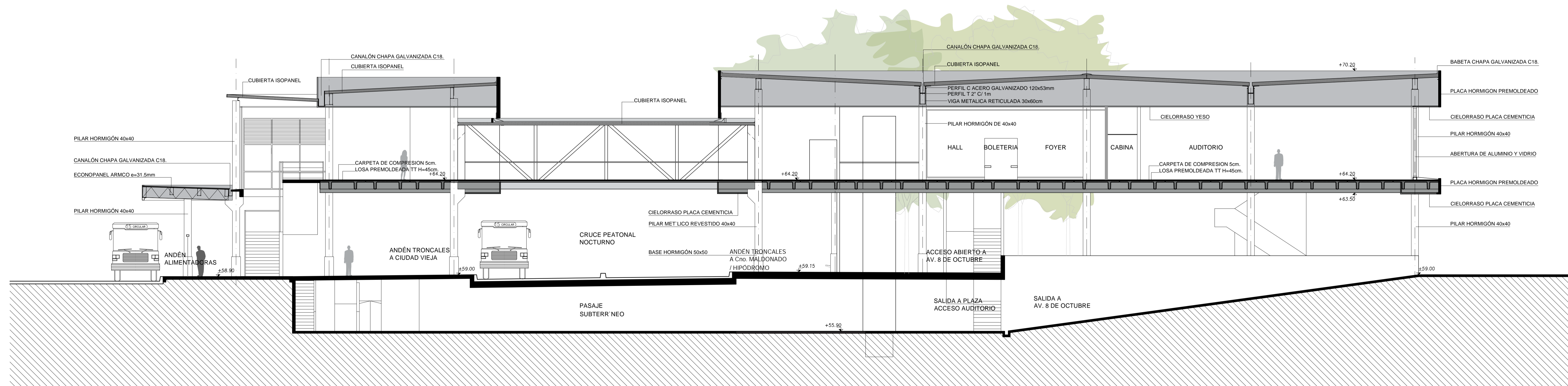
CORTE AA
