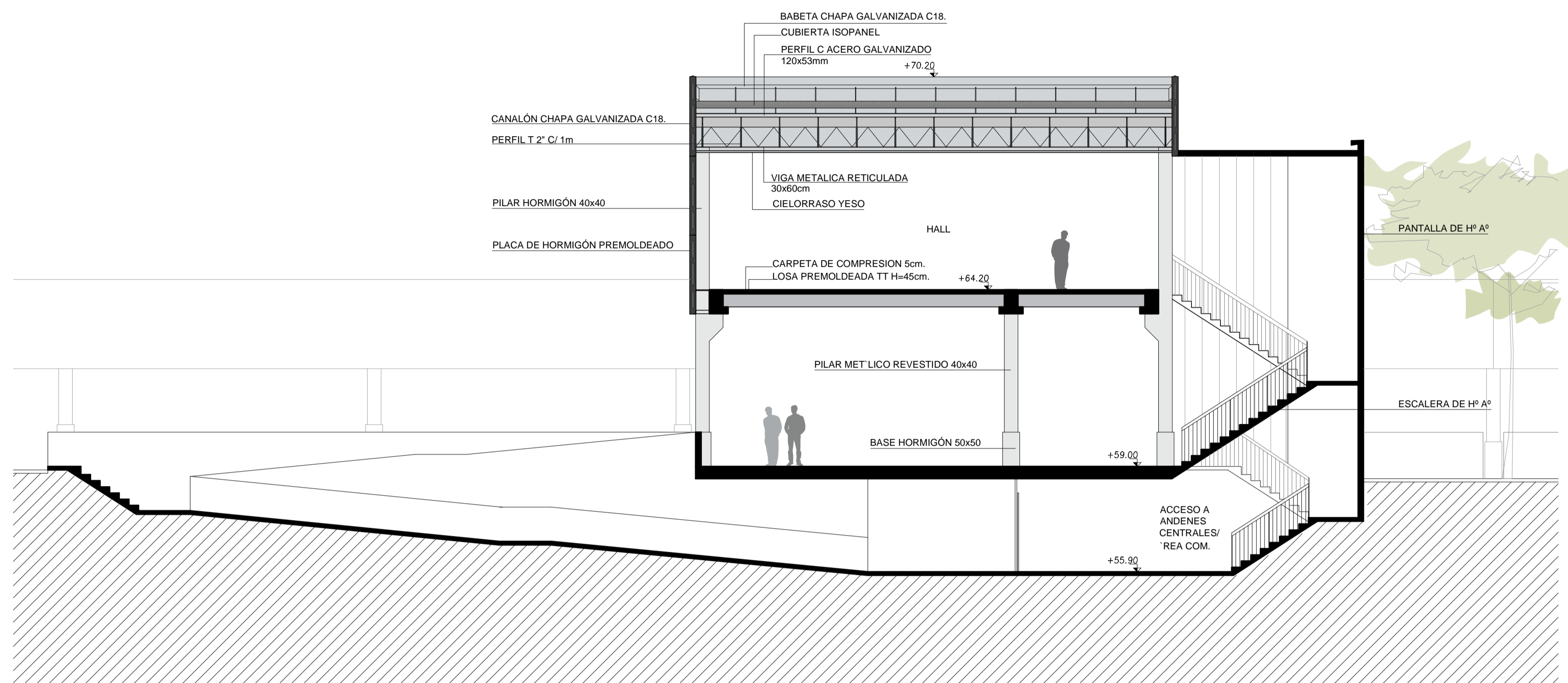
CORTE BB
